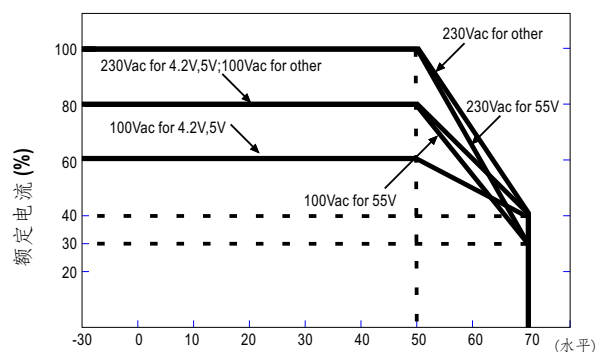
无铅板时环境温度(°C)
